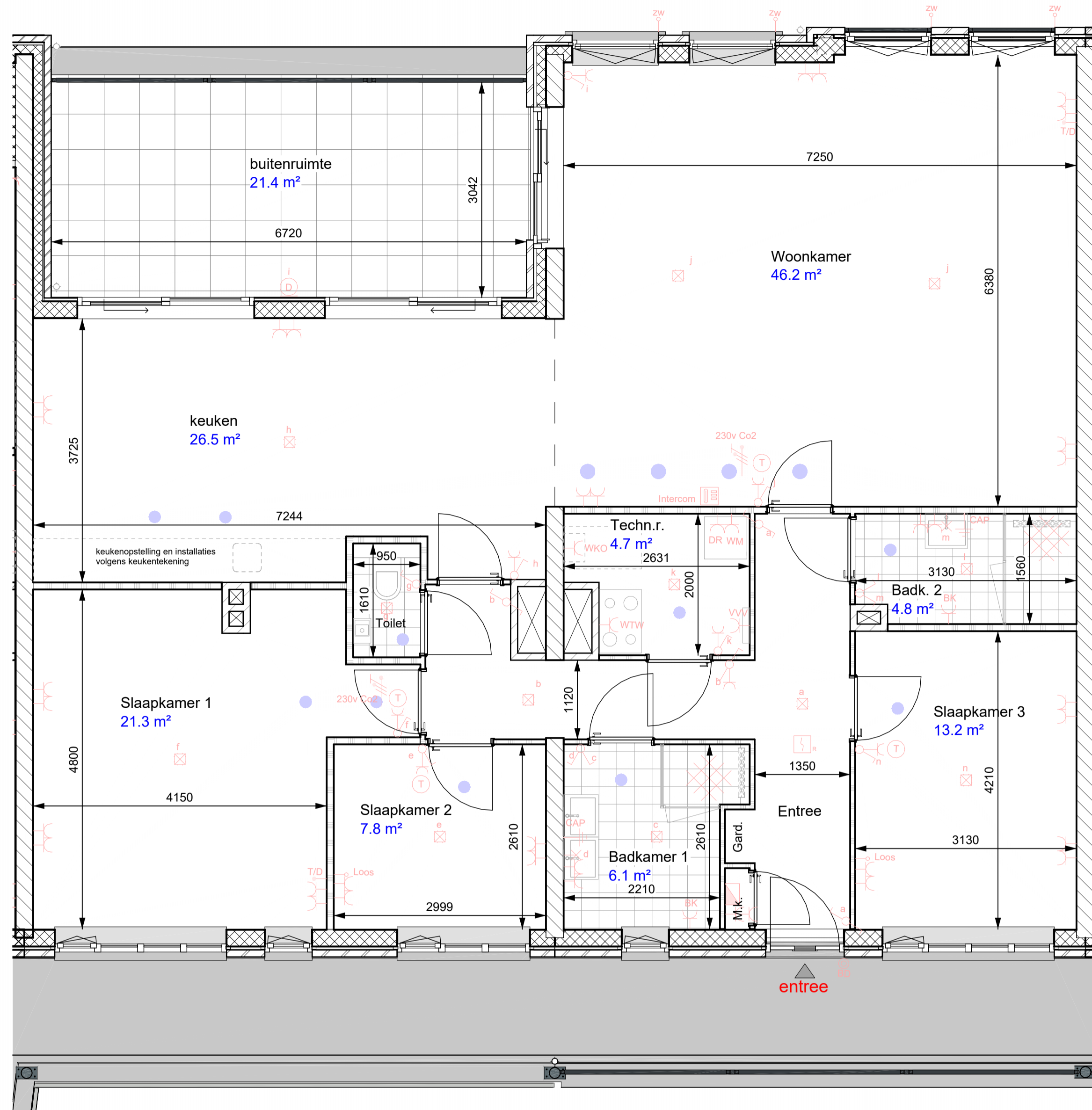
Plattegrond
